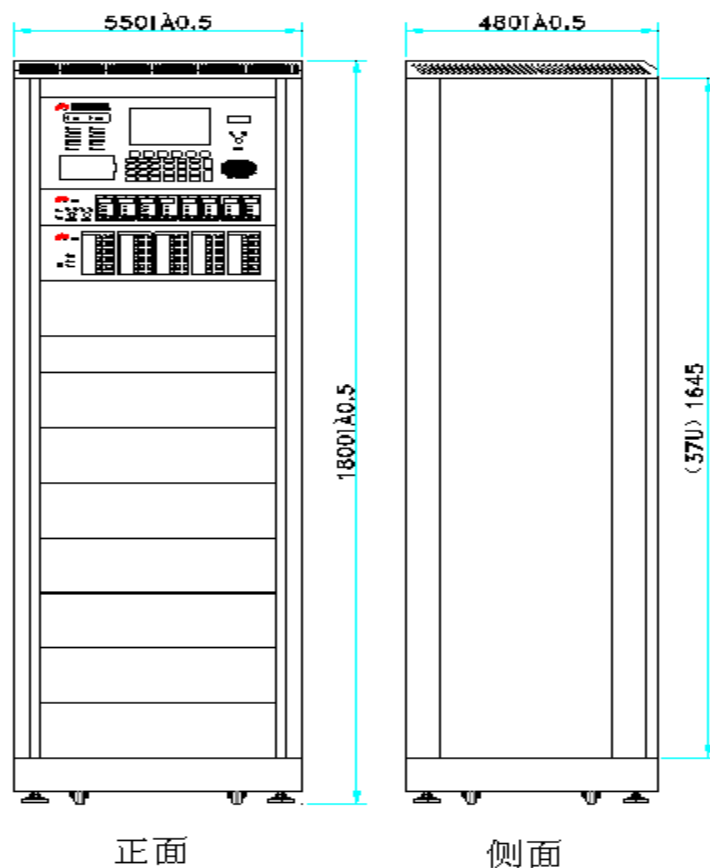
JB-TG-JF999 火灾报警控制器（联动型）外形图：
